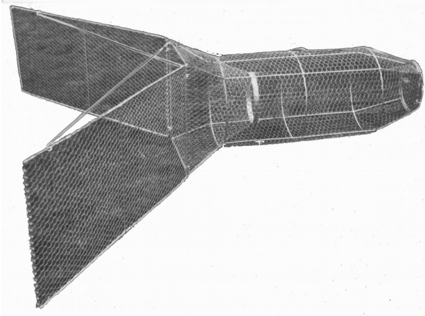
Modell 5/B für den Fang gestellt
